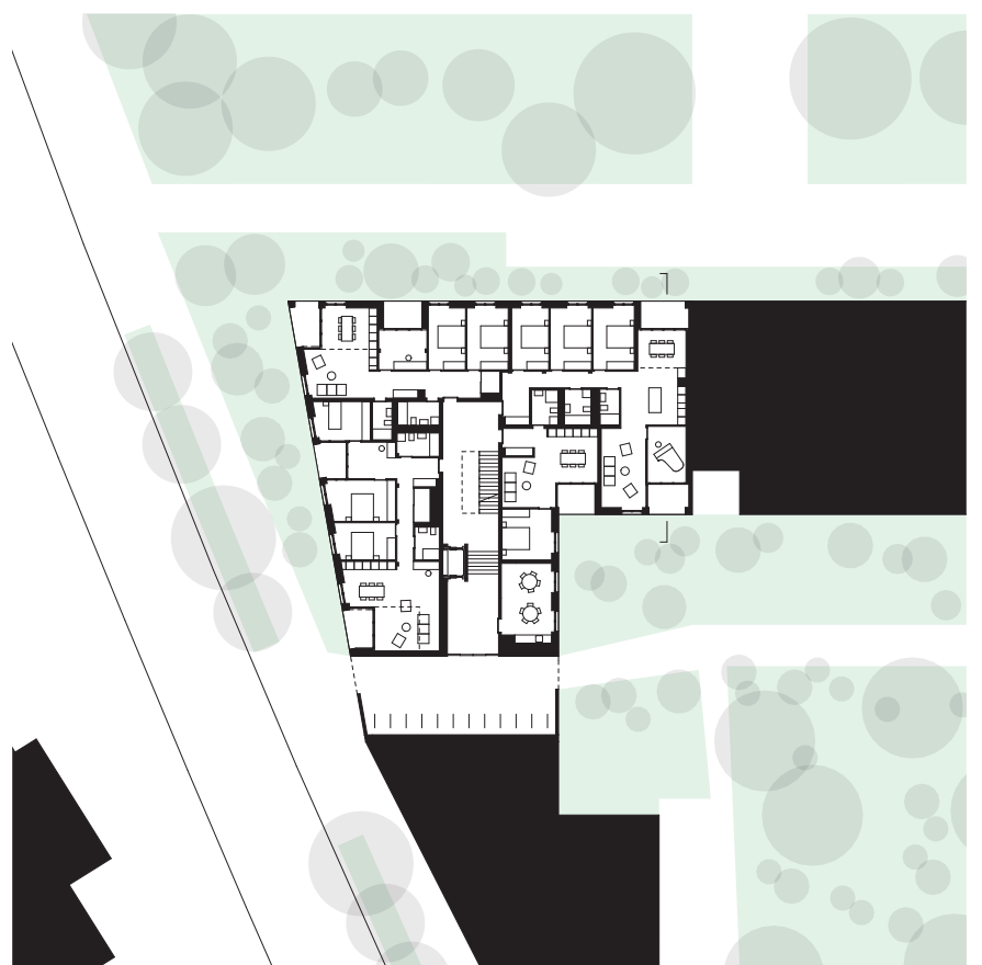
Niv. 0 - Erdgeschoss
